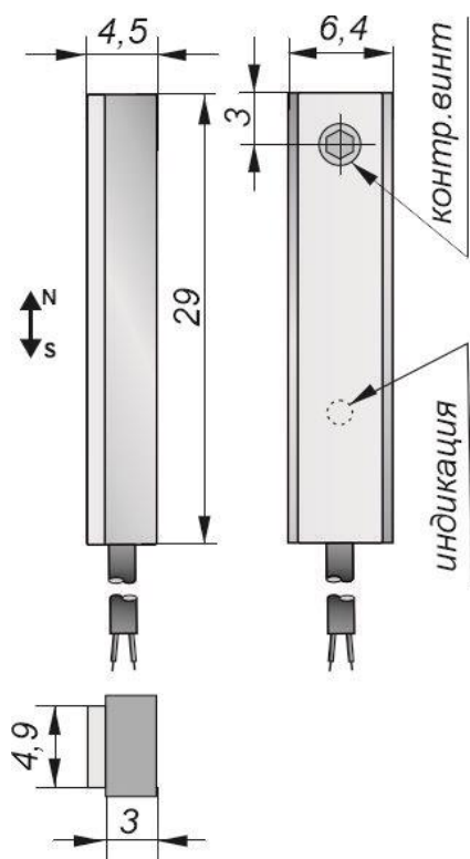
Габаритный чертеж
